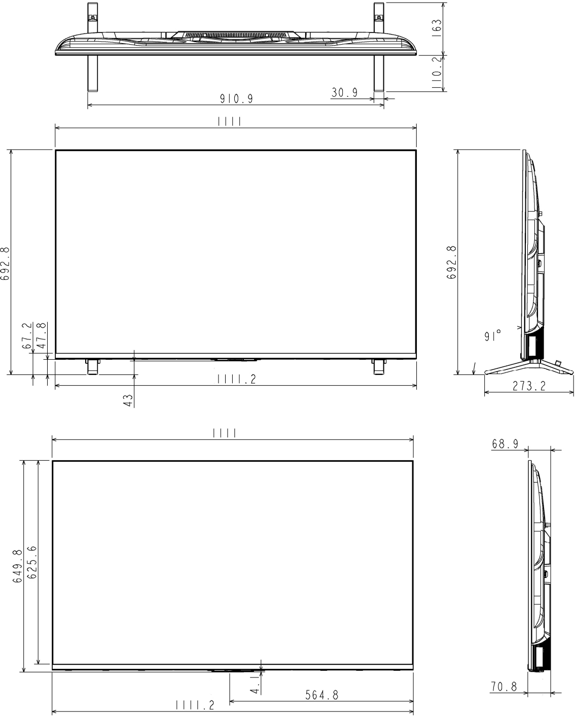
外形図 50E350R
