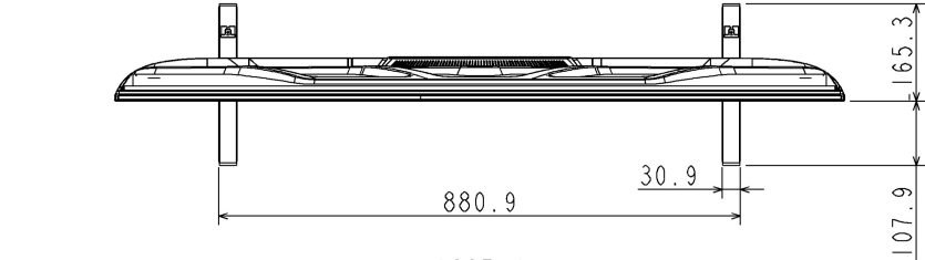
外形図 55E350R
