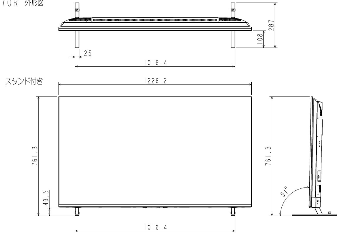
55E670R 外形図
