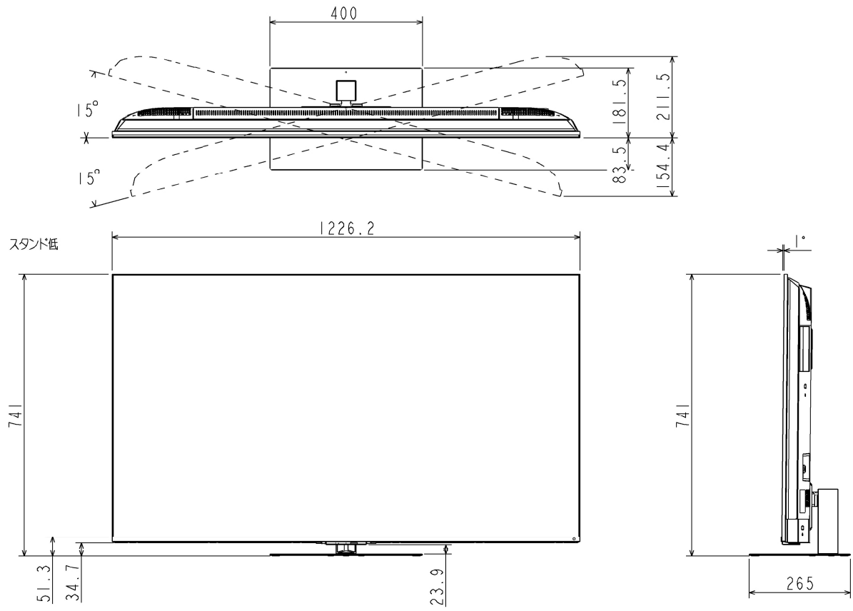
55Z770R 外形図
