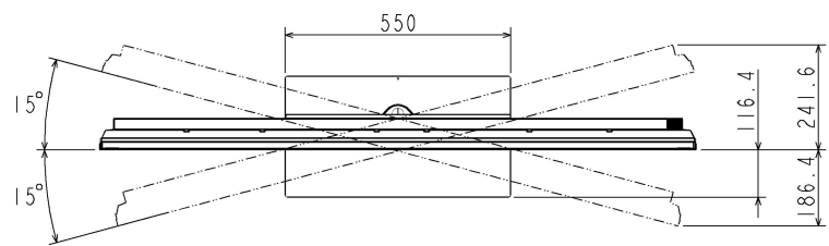
65Z970N 外形図
