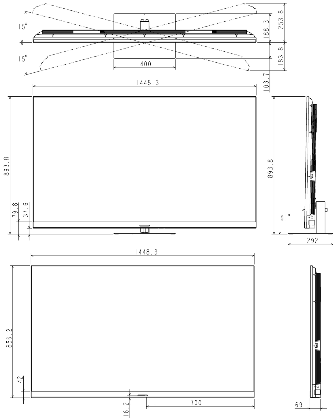
外形図 65Z970R
