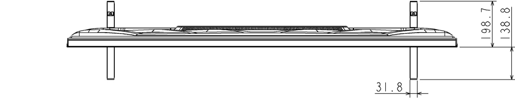
外形図 75E350R
