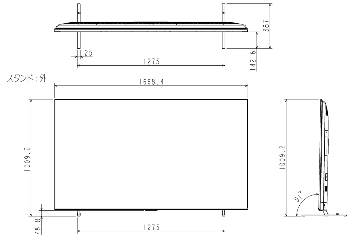
75M550R 外形図
