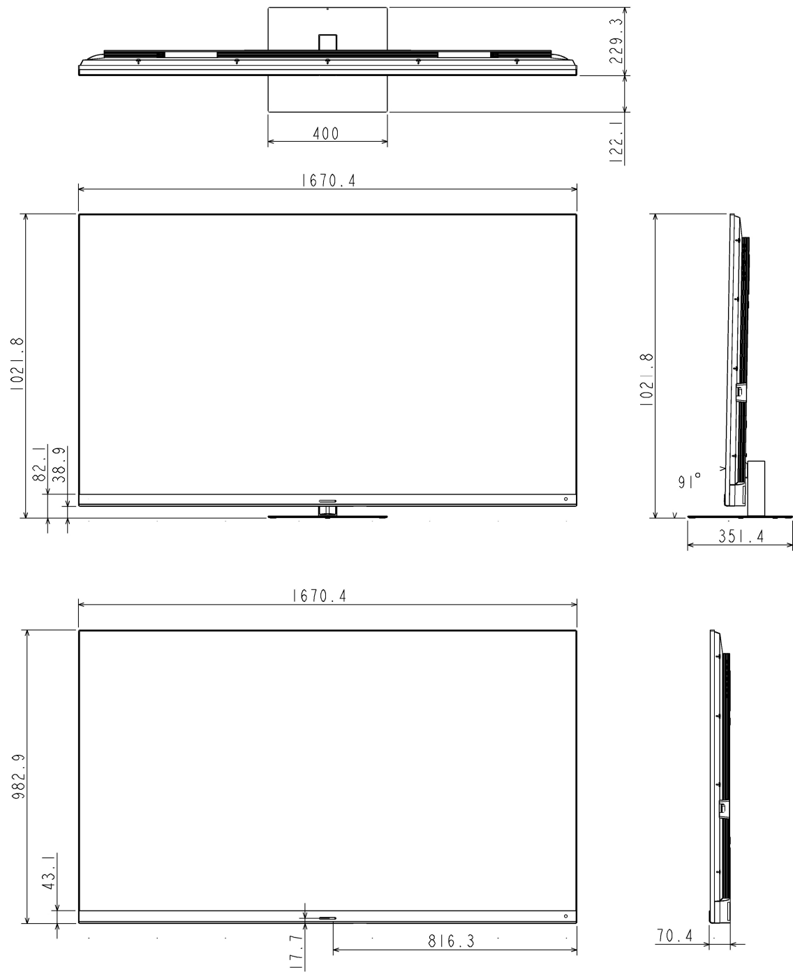
外觀圖 75Z875R
