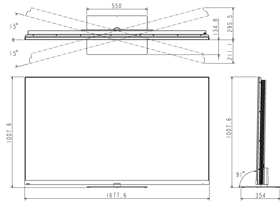
75Z970N 外形図 (rev.01)
