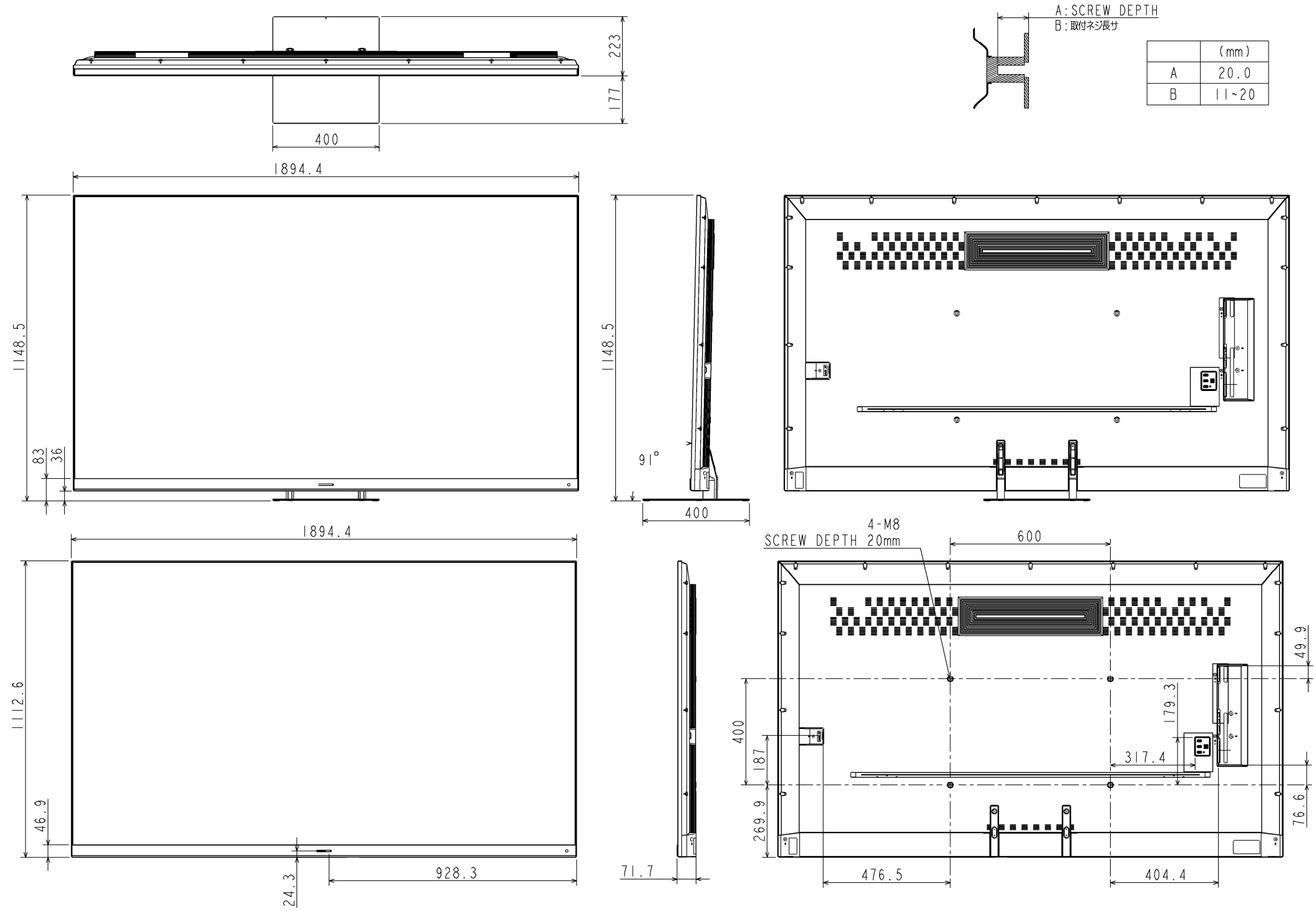
外觀圖 85Z875R
