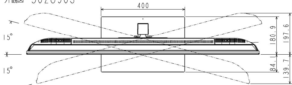
スタンド：低
