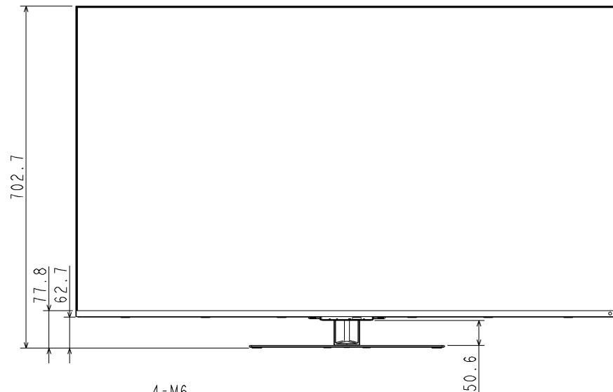
スタンド：高
