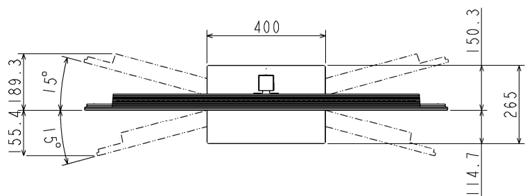
スタンド：低
