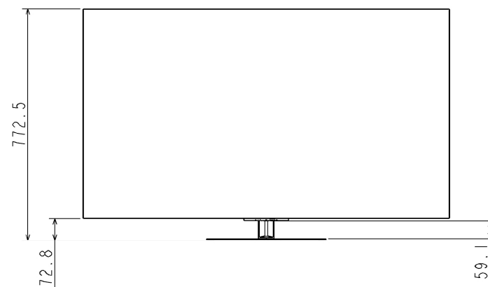
スタンド：高
