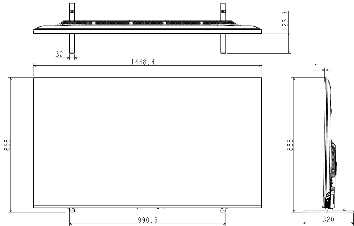
65Z570L 外形图
