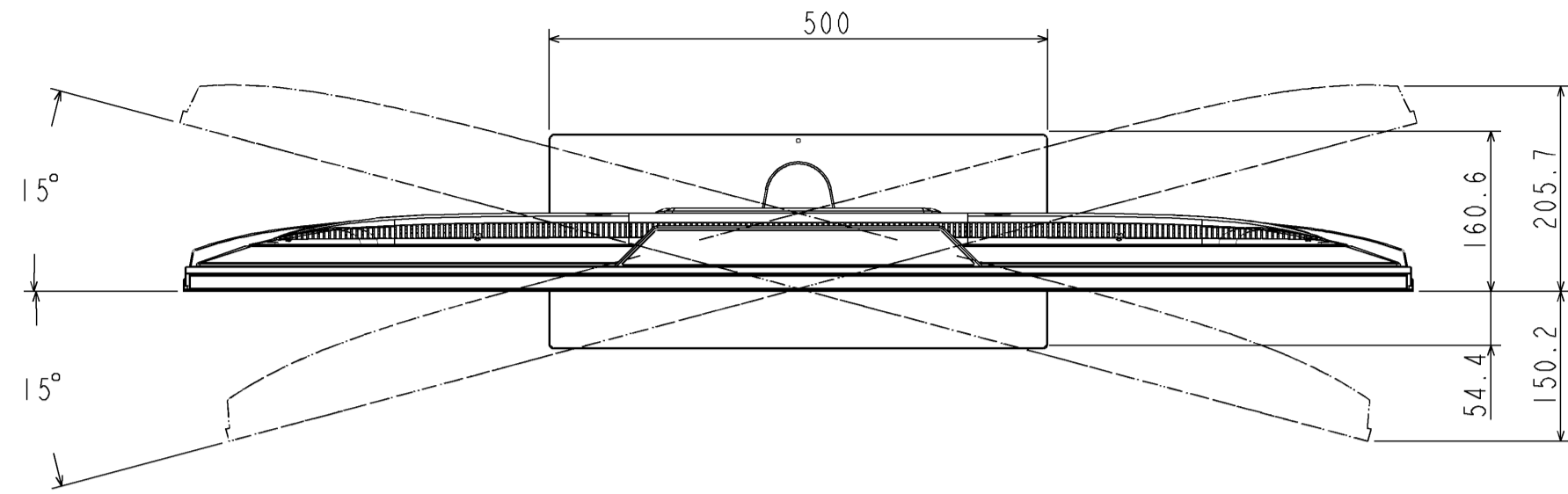
55Z670K 外形圖
